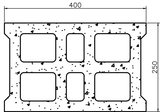
YÜKSEKLİK=200mm HEIGHT=200mm
