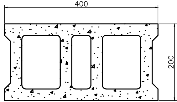
YÜKSEKLİK=200mm HEIGHT=200mm
